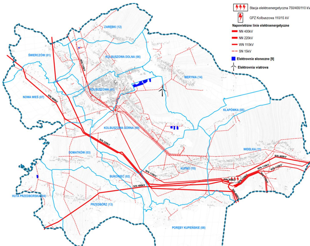
Rys.27.Rozmieszczenie infrastruktury elektroenergetycznej w gminie
